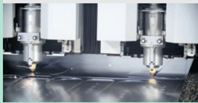
Doppelte Power beim Lasern – Ski-Alu-Sandwichbauteile beim Zuschneiden in einer Zweikopf-Highspeed-Laseranlage
